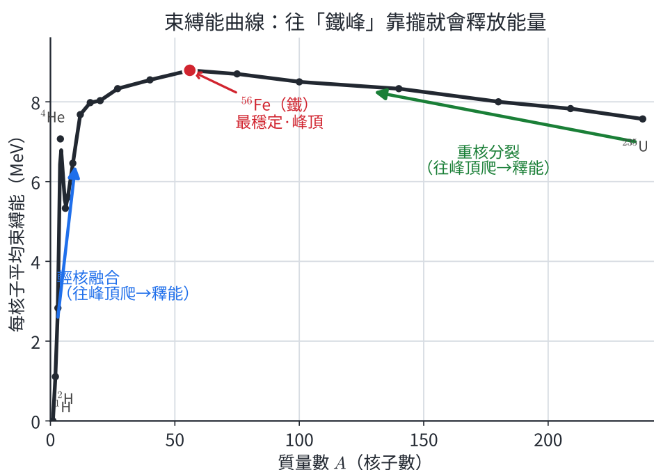
圖 5-3：束縛能曲線。縱軸為每核子平均束縛能、橫軸為質量數 A 。鐵（ ^{56}\text{Fe} ）位於峰頂、最穩定；左側輕核融合、右側重核分裂，都往峰頂靠攏並釋放能量。
