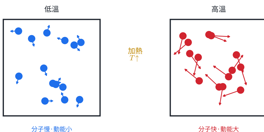
圖 5-4：溫度是分子亂動劇烈程度的量度。左側低溫、分子慢、動能小；右側高溫、分子快、動能大。對理想氣體，內能 \propto T 。
