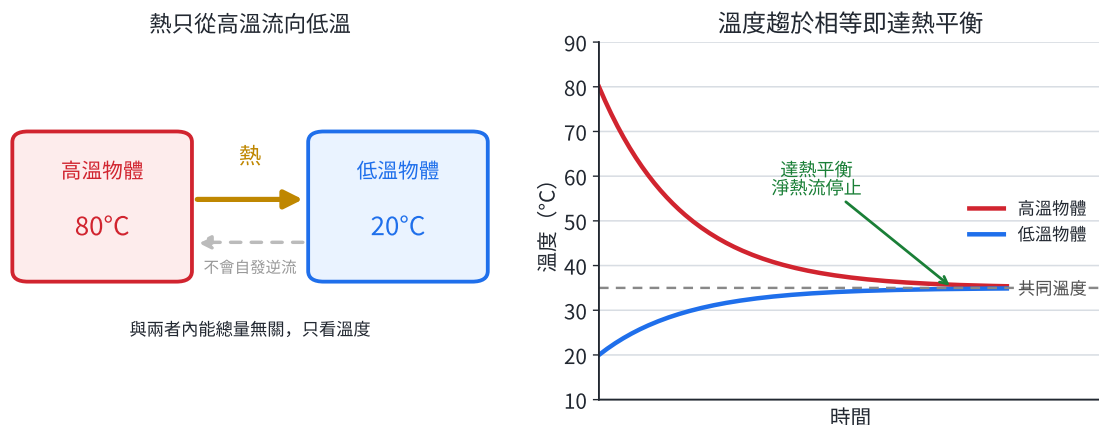
圖 5-5：熱平衡。左——熱只自發地從高溫物體流向低溫物體（不會自發逆流），流向只看溫度、與內能總量無關；右——兩者溫度逐漸趨近，相等時淨熱流停止，即達熱平衡。
