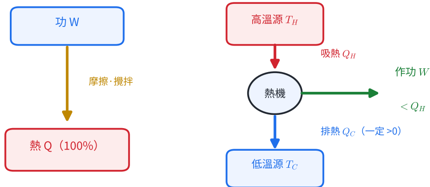
圖 5-7：能量的方向性。左——功可以 100% 變成熱；右——熱機從高溫源吸熱 Q_H 、對外作功 W ，但一定有一部分熱 Q_C 排到低溫源，效率小於 100%。
